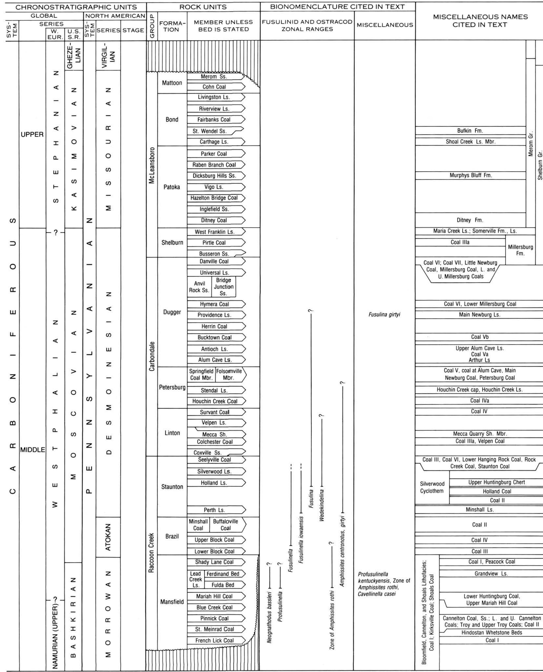
A. PENNSYLVANIAN
