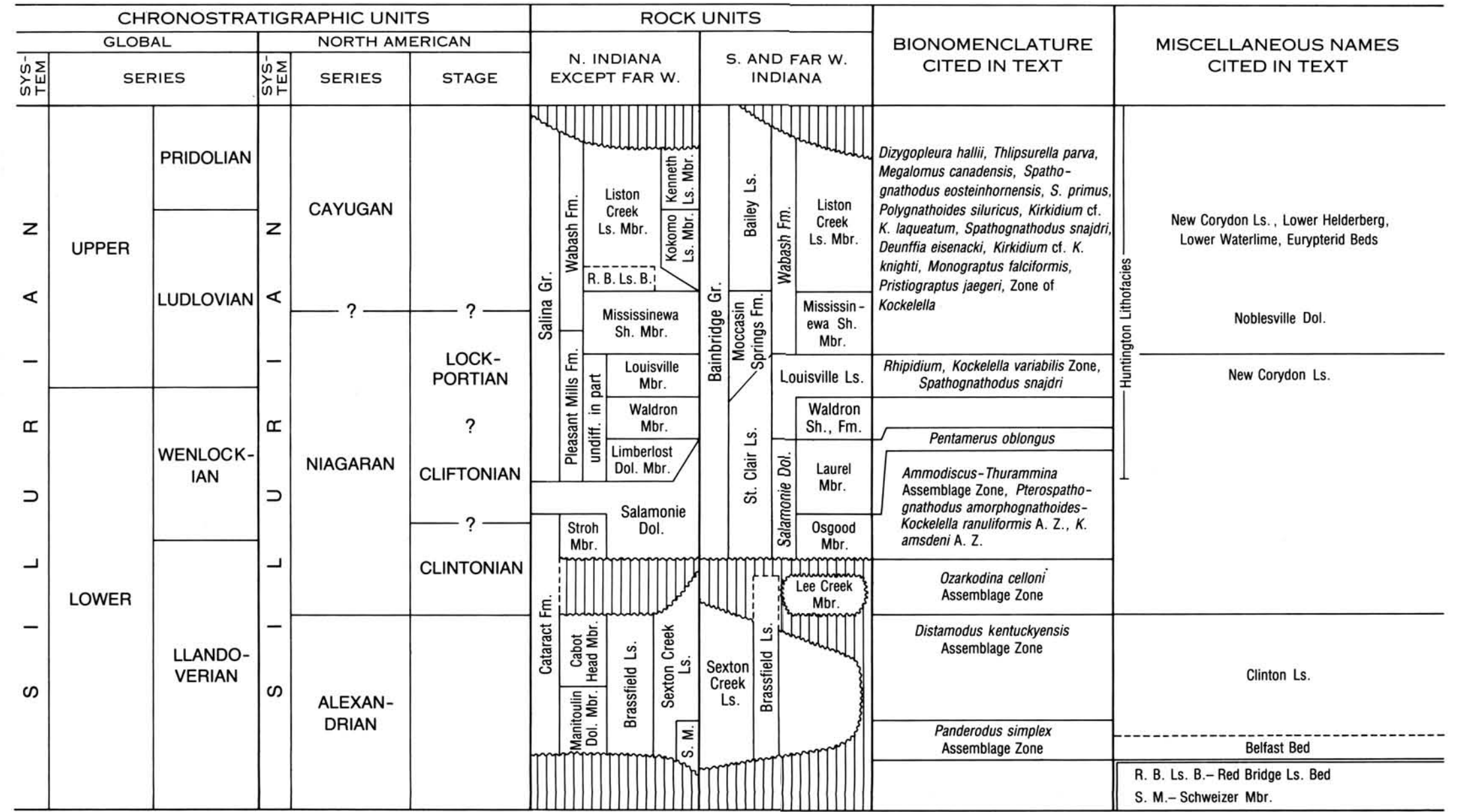
D. SILURIAN
