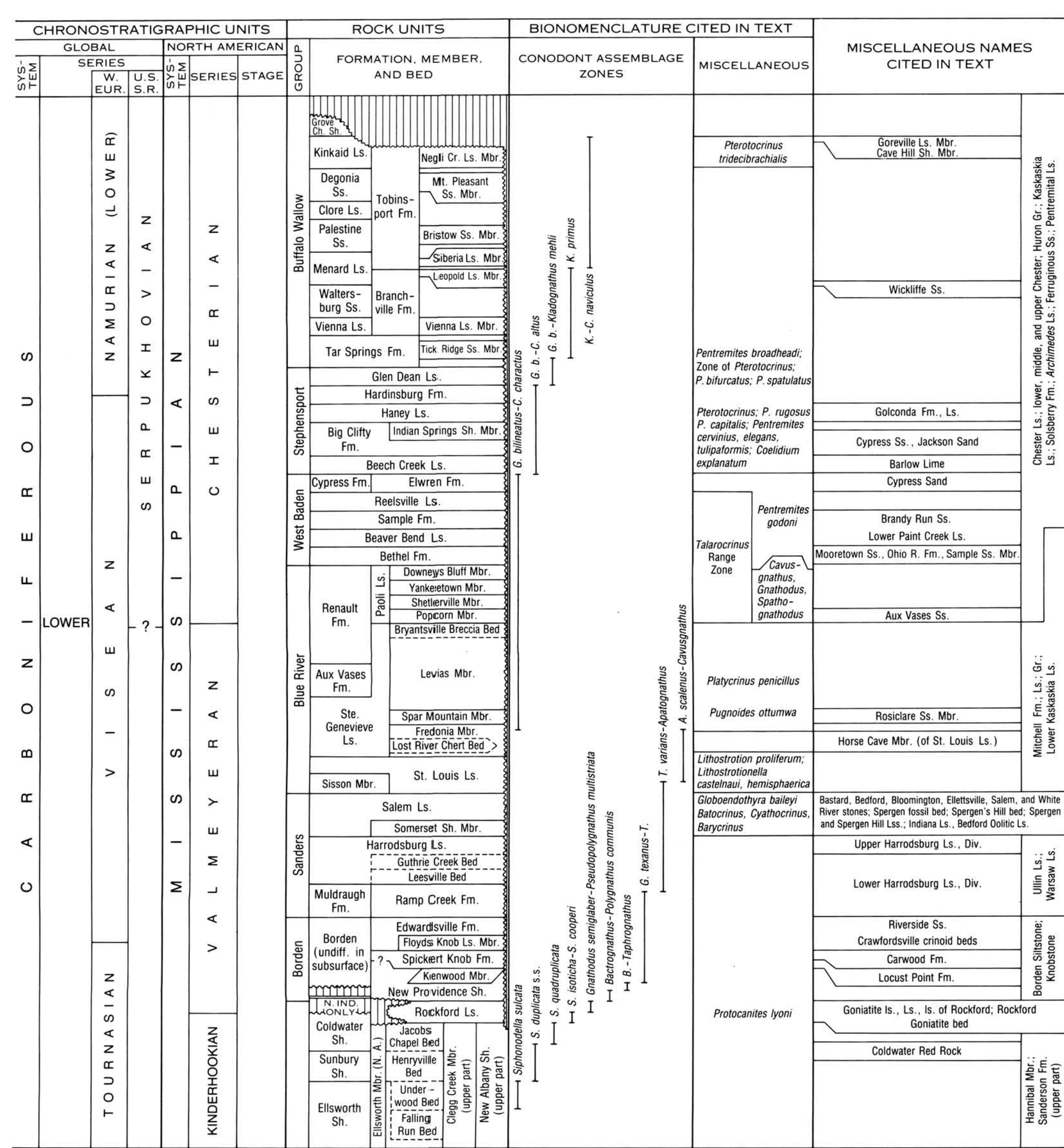
B. MISSISSIPPIAN
